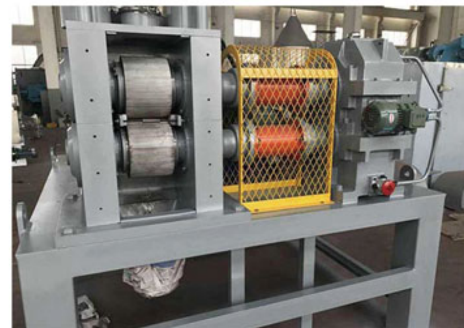
造粒机 Comminutor
